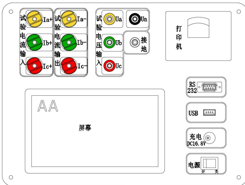
图 2 面板布置图
