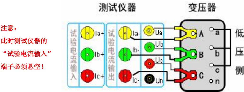
图 22 容量测试及内置三相电源负载测试的接线方法
