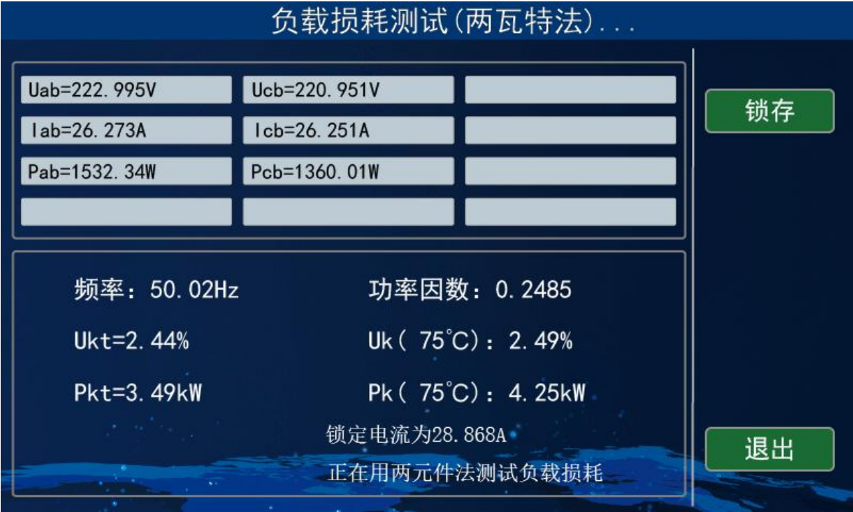
图 14-1 两瓦特法负载损耗测试
