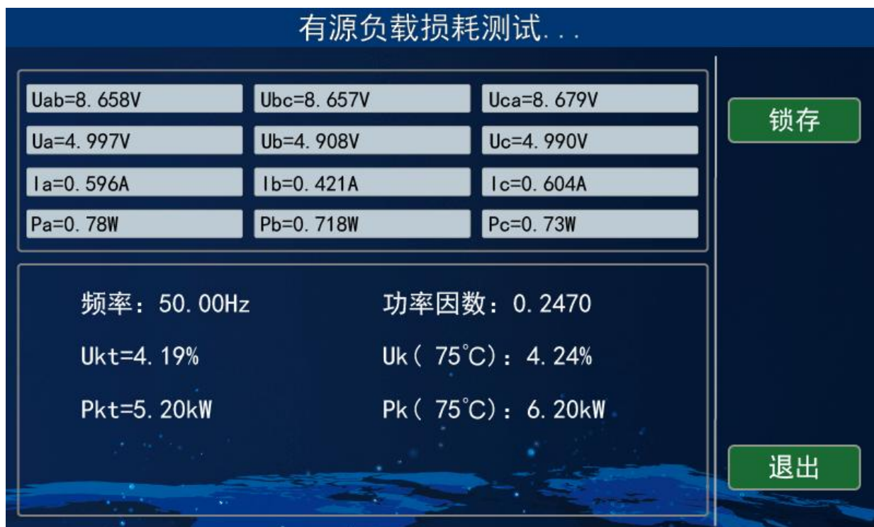
图 15-2 内置三相负载测试结果
