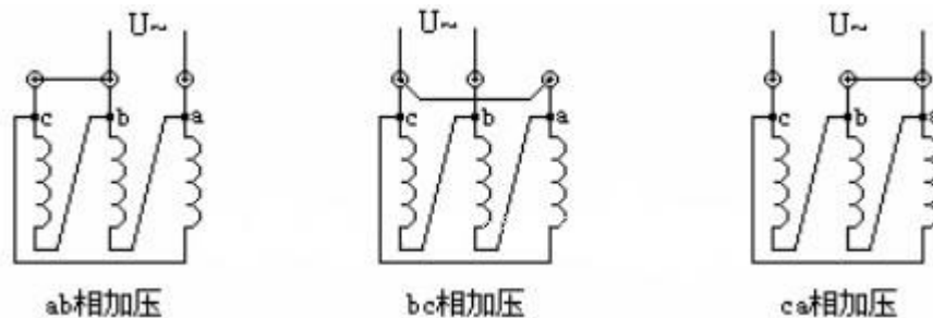
图 26 加压绕组为 \Delta 型连接的接线示意图
