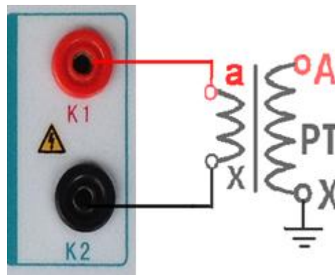
图 29, PT 励磁特性接线图
