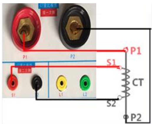
图 13，电流法 CT 变比极性 (角差比差) 接线图
