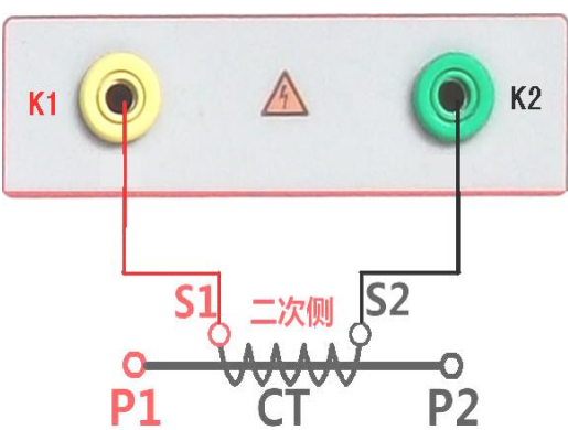
图 5，CT 励磁特性接线图
