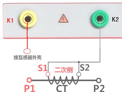
图 20, CT 交流耐压接线图
