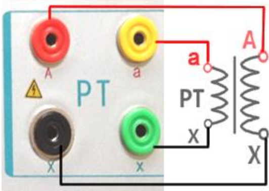
图 31，PT 变比极性（角差比差）接线图
