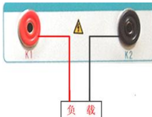
图 22, CT 二次负荷接线图
