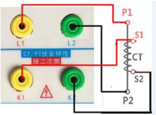
图 27 综合测试接线图
