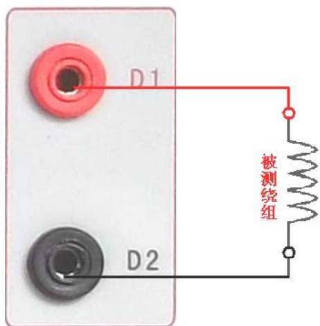
图 25，直阻测试接线图
